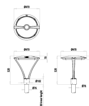
ON POLE Ø76
