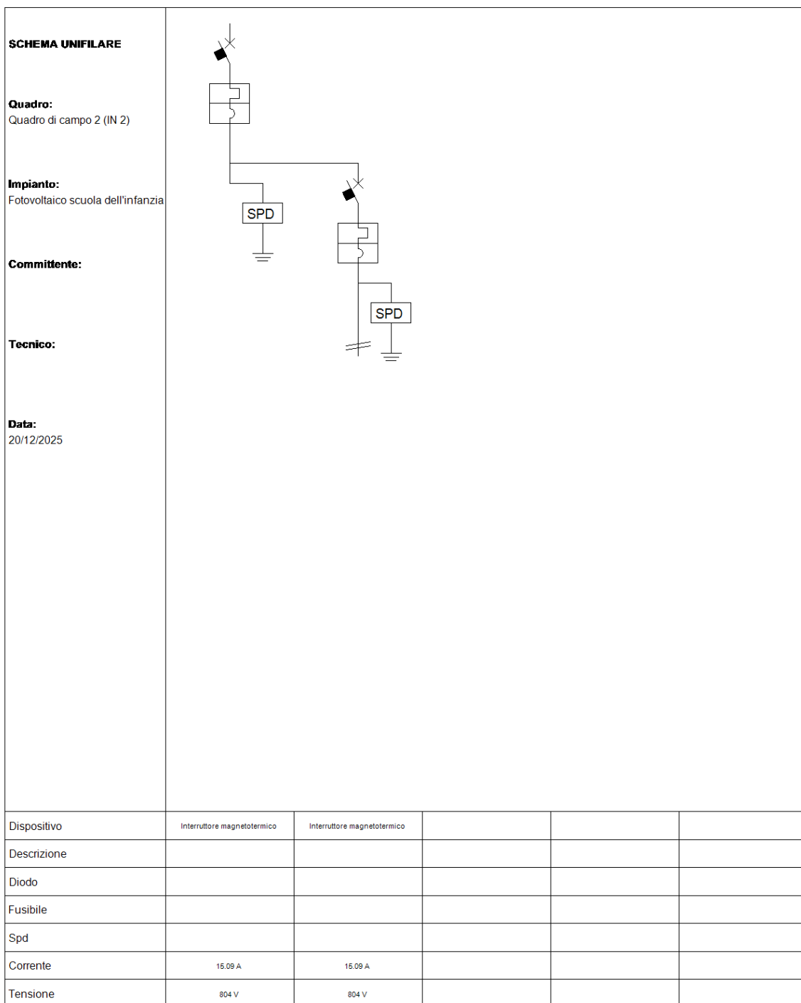
Fig. 8: Schema unifilare quadro "Quadro di campo 2"
