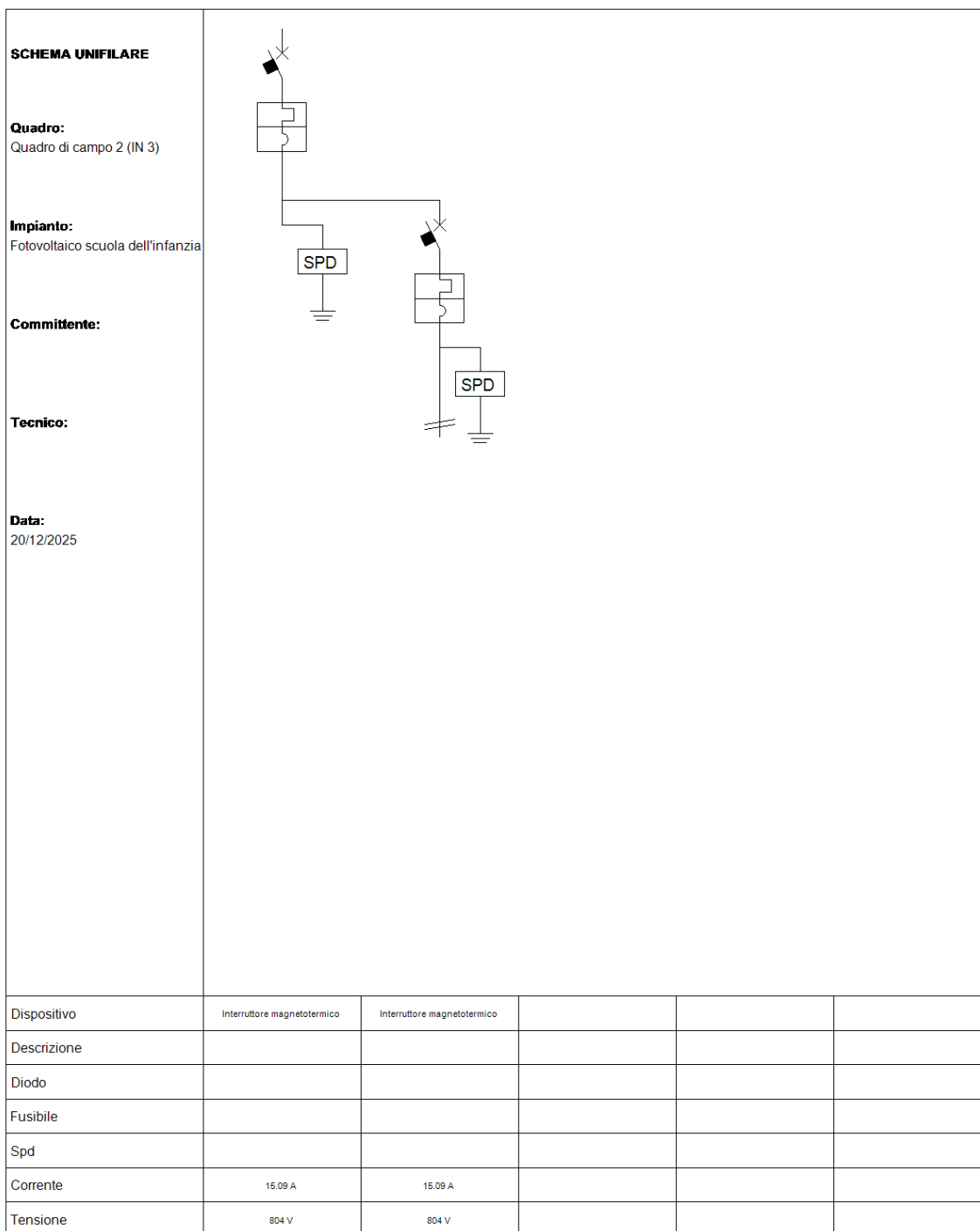
Fig. 9: Schema unifilare quadro "Quadro di campo 2"
