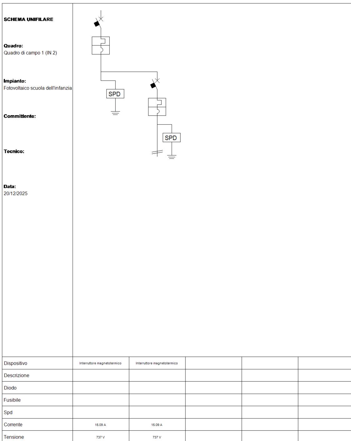
Fig. 12: Schema unifilare quadro "Quadro di campo 1"
