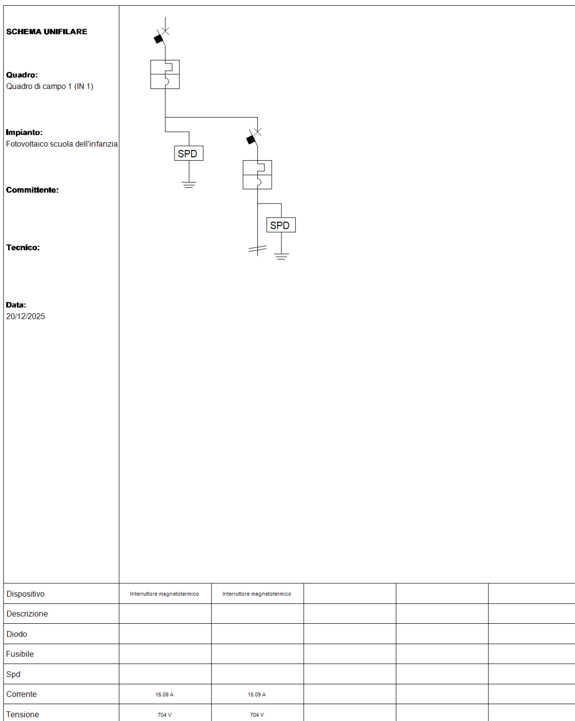
Fig. 11: Schema unifilare quadro "Quadro di campo 1"
