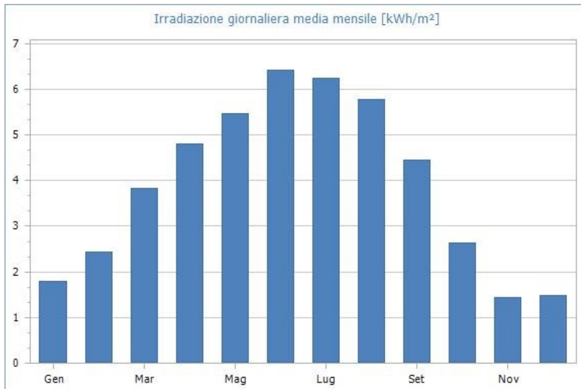
Fig. 1: Irradiazione giornaliera media mensile sul piano orizzontale [kWh/m 2 ]- Fonte dati: UNI 10349:2016 - Stazione di rilevazione: Iglesias
