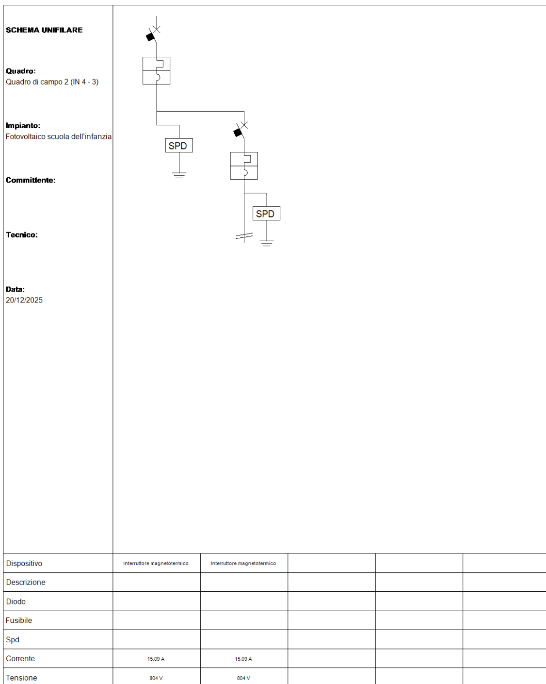
Fig. 10: Schema unifilare quadro "Quadro di campo 2"
