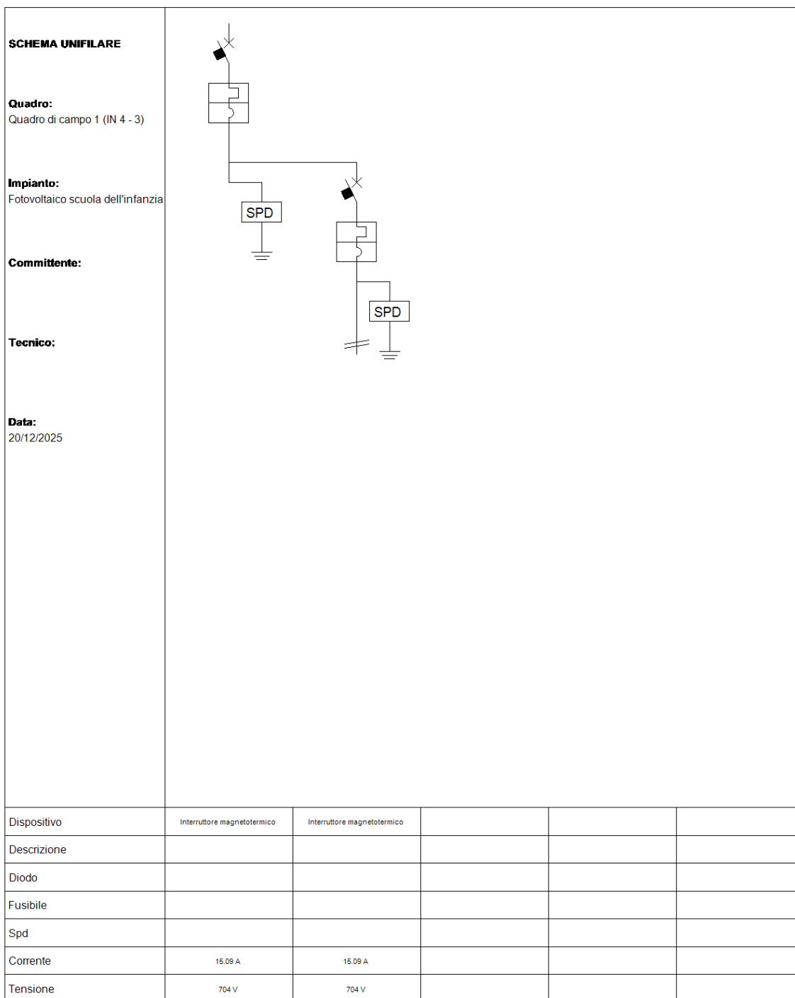
Fig. 14: Schema unifilare quadro "Quadro di campo 1"
