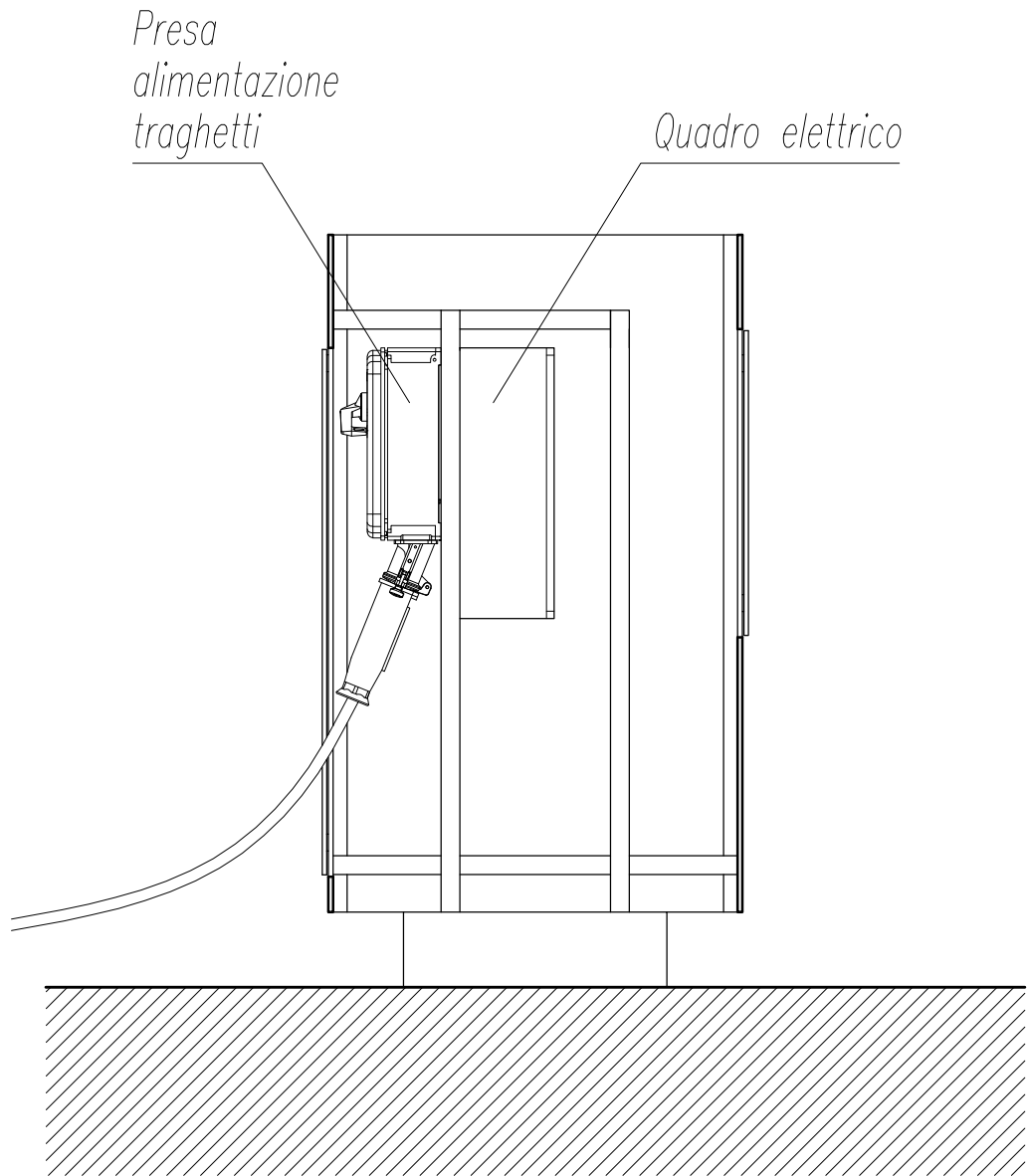
Sezione CC'
